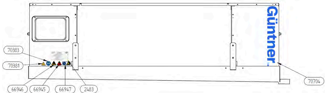
Vue de côté (câblage à droite)
