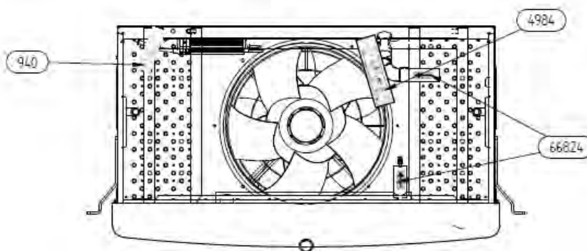
Vue côté entrée d'air derrière la grille de protection (côté tuyauterie)
